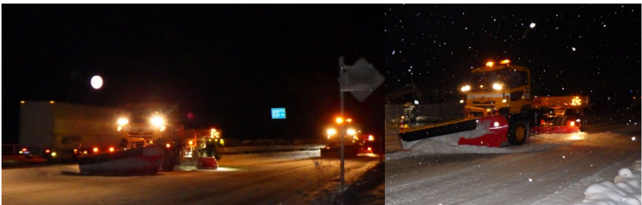
暴風雪(令和5年1月23日～)の影響により夜を徹した国道8号の除雪作業 (一社) 富山県建設業協会
