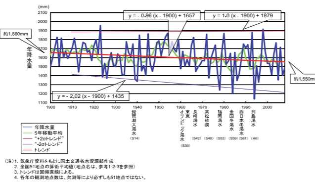
図-4 日本の年降水量の経年変化
