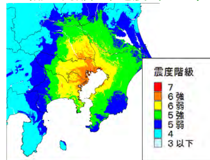
首都直下地震震度分布 (都心南部直下地震 (M7.3))
