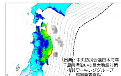
日本海溝沿い巨大地震震度分布
